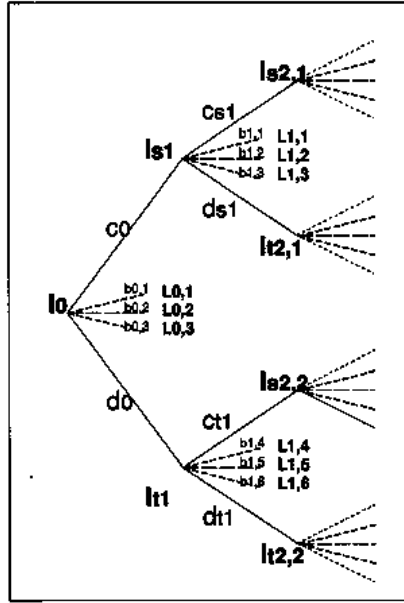
Figure 54 Arbre des rayons issus d'un pixel
