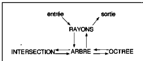
Figure 28 Traitement coopératif de 4 tâches
