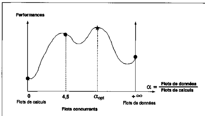
Figure 85 Etude des performances de l'algorithme à flots concurrents en fonction du rapport entre le nombre de messages d'envoi de données et le nombre de messages d'envoi de calculs.
