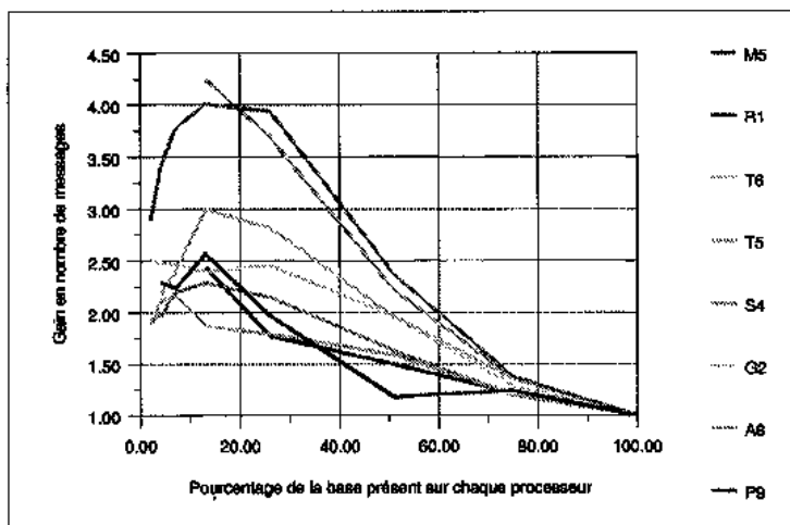
Figure 75 Gain en nombre de messages de l'algorithme à flux multi-informatifs par rapport à l'algorithme à flux de données
