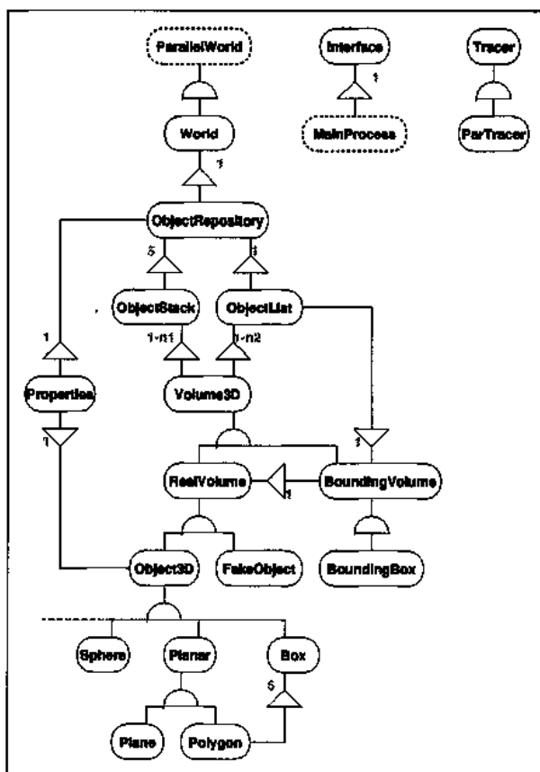
Figure 106 Diagramme objet du moteur d'intersection
