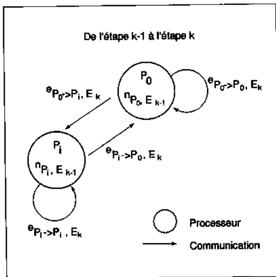
Figure 43 Schéma du modèle
