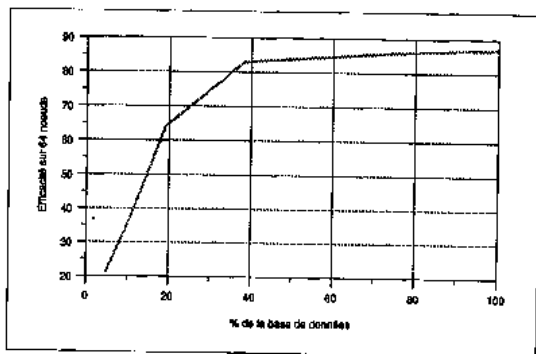
Figure 39 Mesures d'efficacité pour 64 processeurs données par Badouel pour l'image Mountain en fonction de la taille mémoire disponible pour chaque processeur
