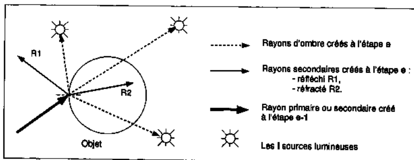
Figure 55 Création de rayons à chaque étape
