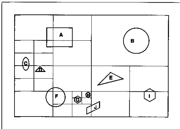
Figure 10 Découpage en quadtree d'une scène 2D
