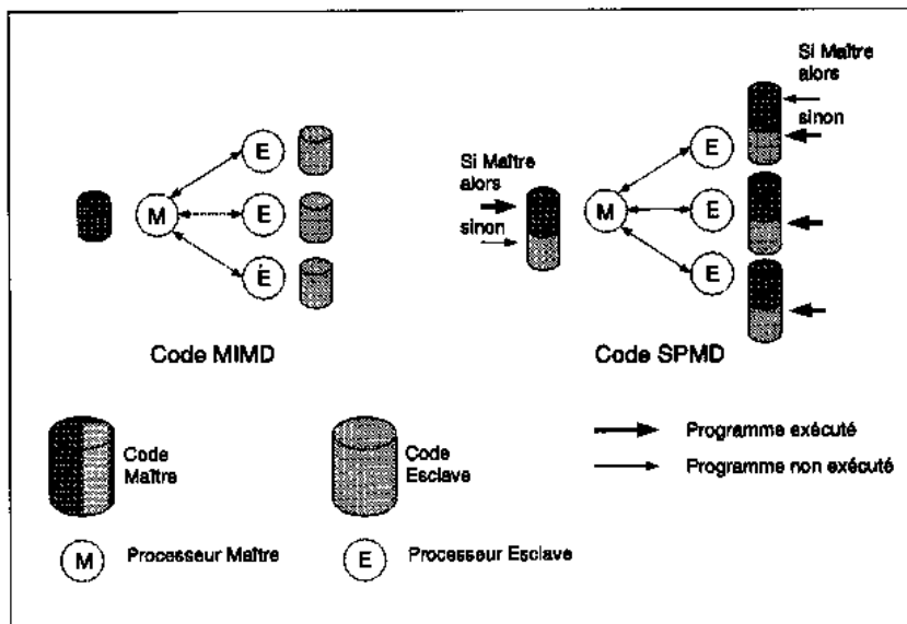
Figure 23 Différences entre codes MIMD et SPMD
