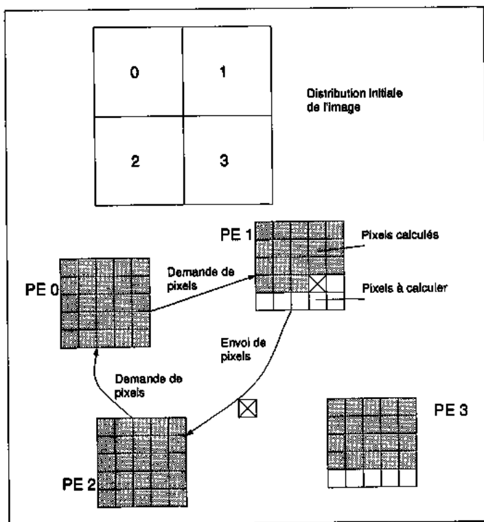
Figure 27 Distribution statique par blocs des pixels et équilibrage dynamique en anneau
