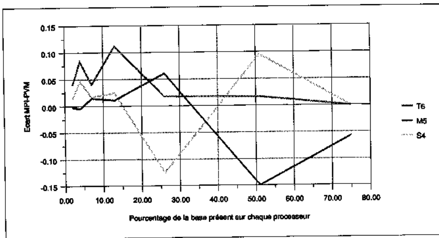
Figure 86 Ecart entre les temps de calculs avec MPI et PVM pour 64 processeurs
