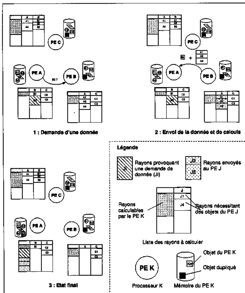
Figure 46 Schéma représentant l'envoi d'un message multi-informatif
