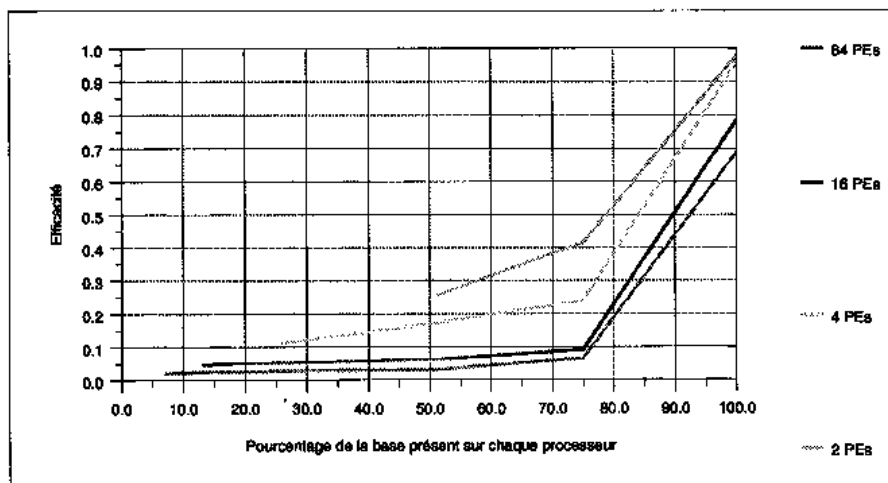
Figure 71 Efficacité pour l'image T5
