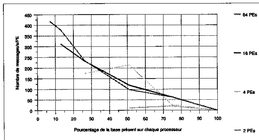
Figure 72 Nombre de messages
