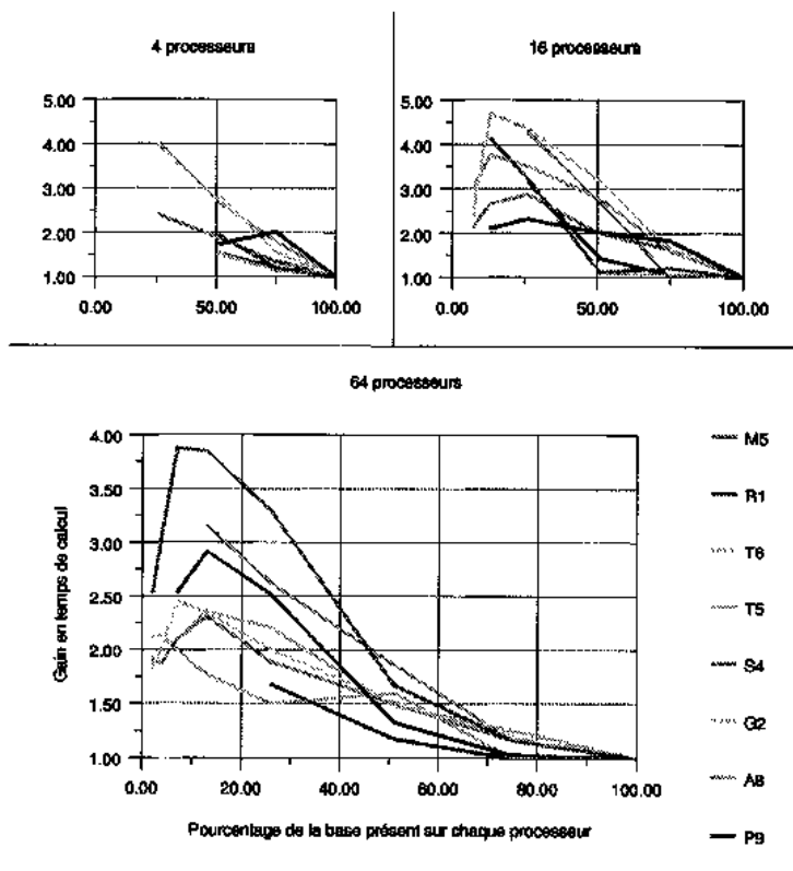
Figure 78 Gains en temps de l'algorithme à flots concurrents par rapport à l'algorithme à flots de données
