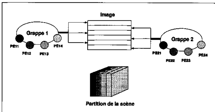
Figure 34 Architecture de la 'parallélisation hybride'
