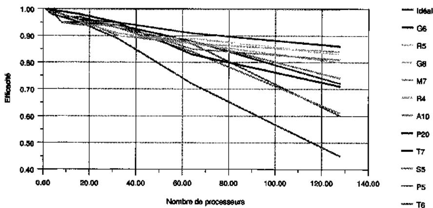
Figure 60 Efficacité avec base dupliquée
