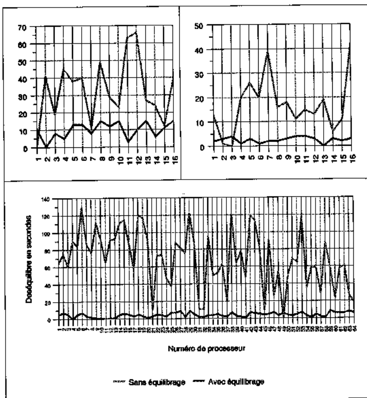
Figure 69 Ré-équilibrage de la charge de chaque processeur
