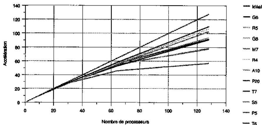
Figure 59 Accélération avec base dupliquée
