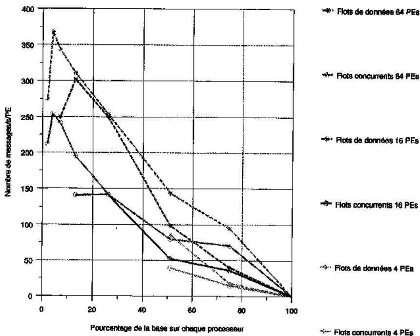
Figure 81 Comparaison du nombre de messages par seconde de l'algorithme à flots concurrents et de l'algorithme à flots de données pour l'image M5
