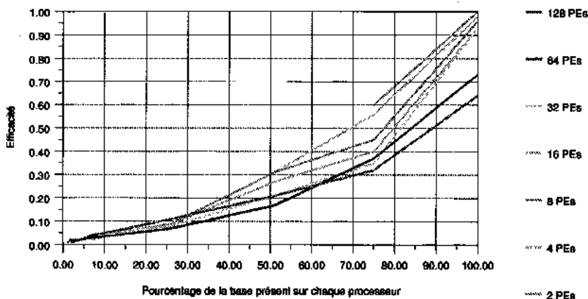
Figure 63 Efficacité en fonction de la distribution de la scène pour l'image M5.
