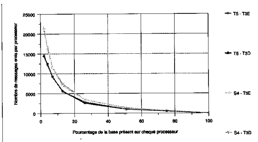
Figure 89 Nombre de messages émis sur CRAY T3D et T3E avec 64 processeurs
