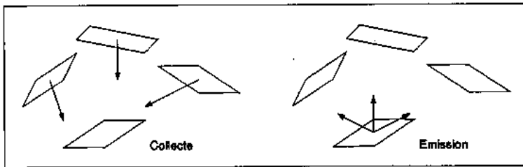
Figure 41 Radiosit  par collecte et par  mission
