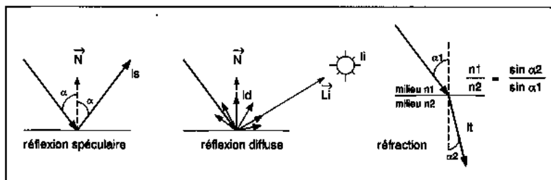
Figure 3 Réflexions et réfraction
