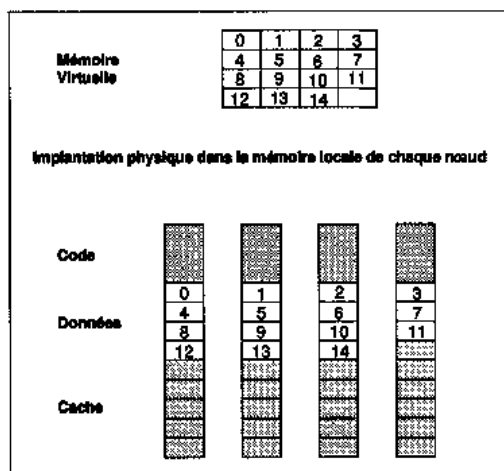
Figure 38 Implantation d'un mémoire partagée virtuelle
