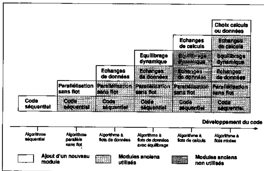
Figure 48 Etapes de développement de l'algorithme parallèle
