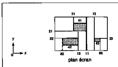
Figure 15 Partition du plan écran
