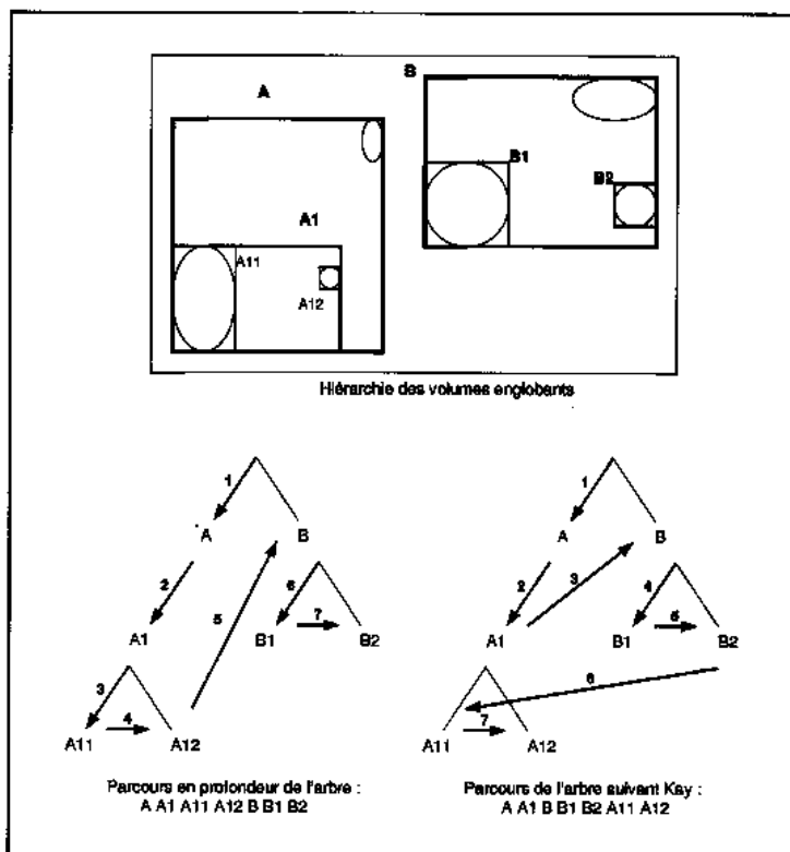
Figure 9 Accélération du parcours d'un arbre
