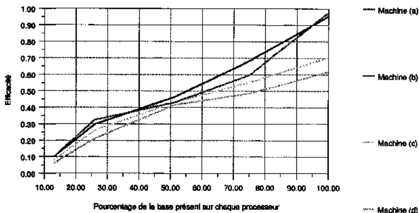
Figure 94 Efficacité des différentes machines
