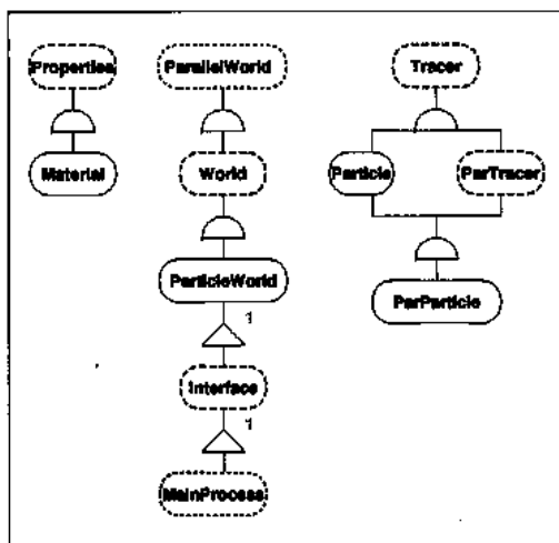
Figure 108 Diagramme objet du module particulaire
