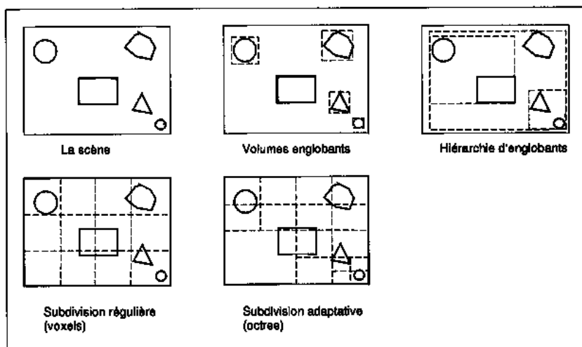
Figure 21 Les types d'accélération séquentielle les plus performants
