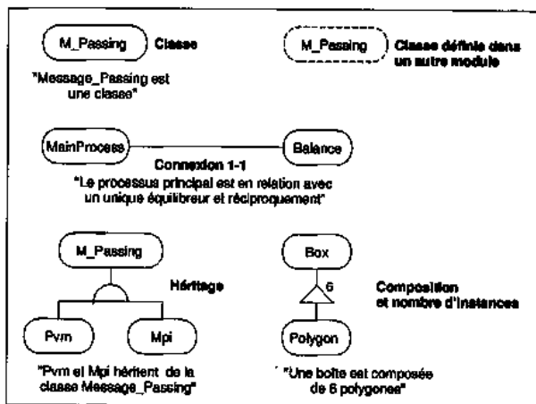
Figure 104. Conventions graphiques de représentation des diagrammes objets
