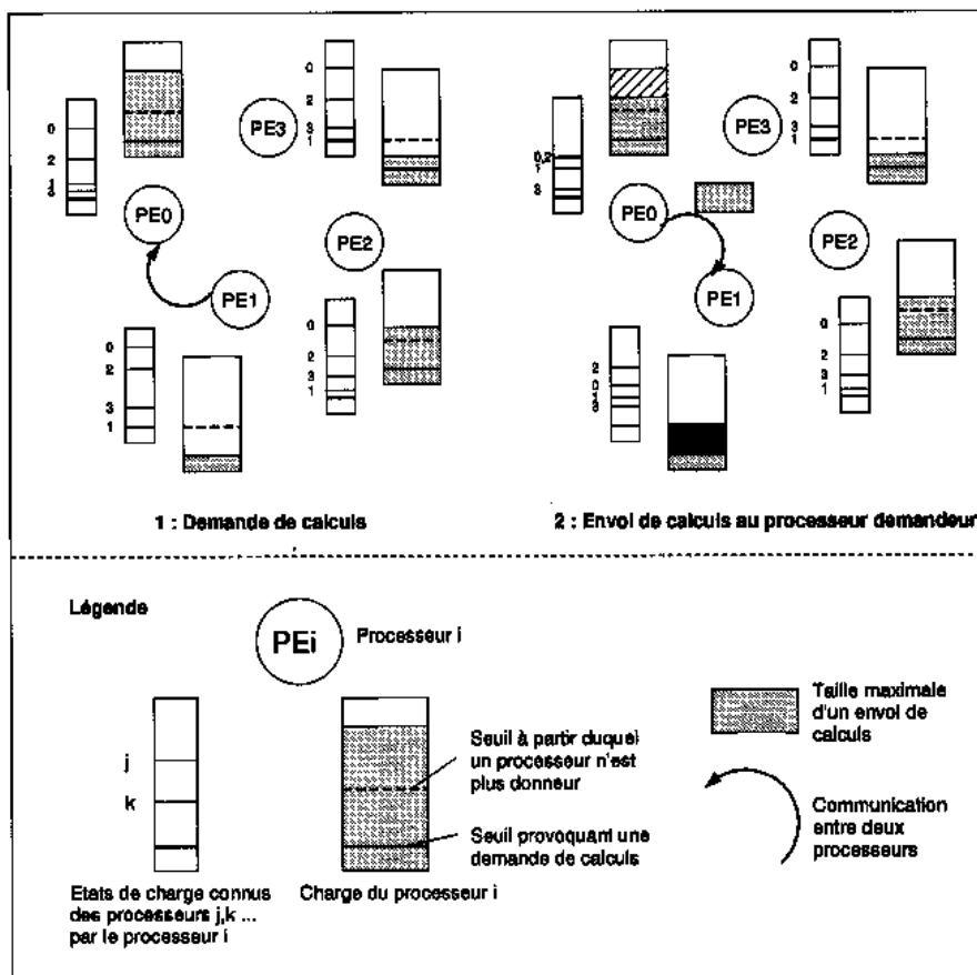
Figure 47 Nouvel équilibrage dynamique
