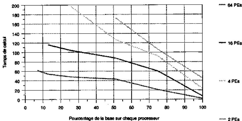
Figure 70 Temps de calcul pour l'image T5
