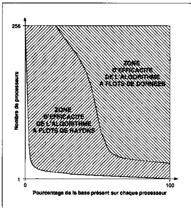
Figure 44 Zones d'efficacité des deux modèles
