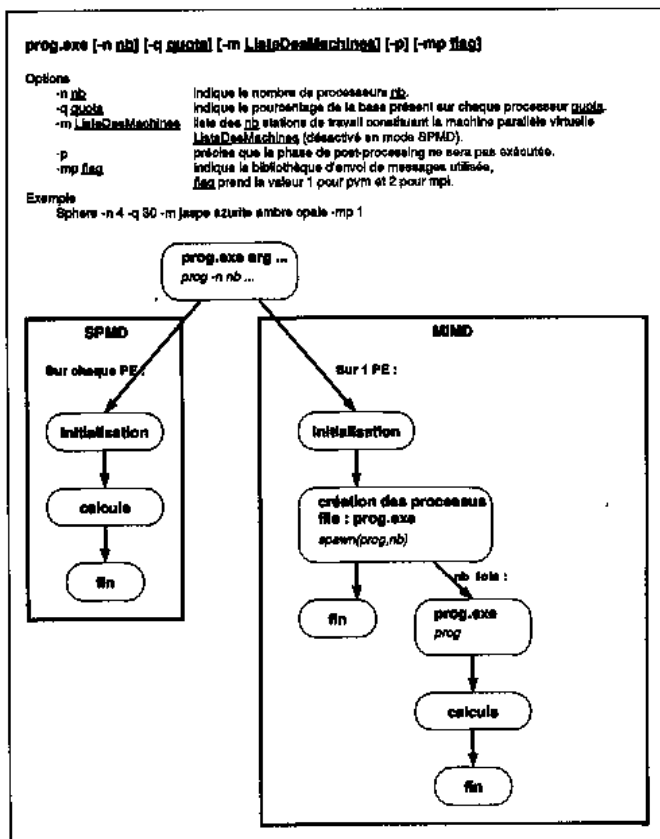
Figure 58 Procédure de lancement du logiciel
