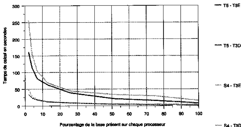
Figure 37 Comparaison des temps de calcul obtenus sur CRAY T3D et T3E avec 64 processeurs
