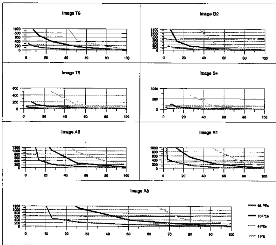
Figure 61 Temps de calcul en fonction de la distribution de la scène pour des images différentes pour des nombres de processeurs différents
