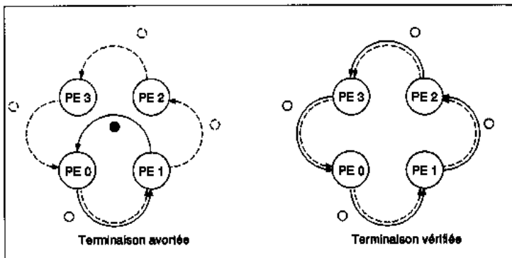
Figure 57 Trajets du jeton sur plusieurs parcours
