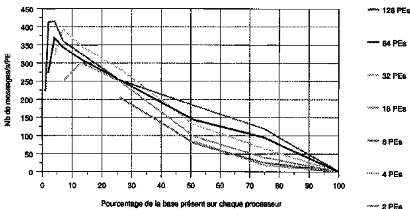
Figure 65 Nombre moyen de messages émis par PE par seconde pour M5
