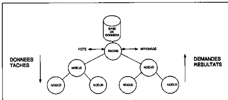
Figure 37 Architecture en forme d'arbre
