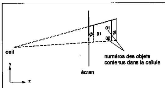
Figure 16 Obtention d'une cellule 3D à partir d'un rectangle de projection
