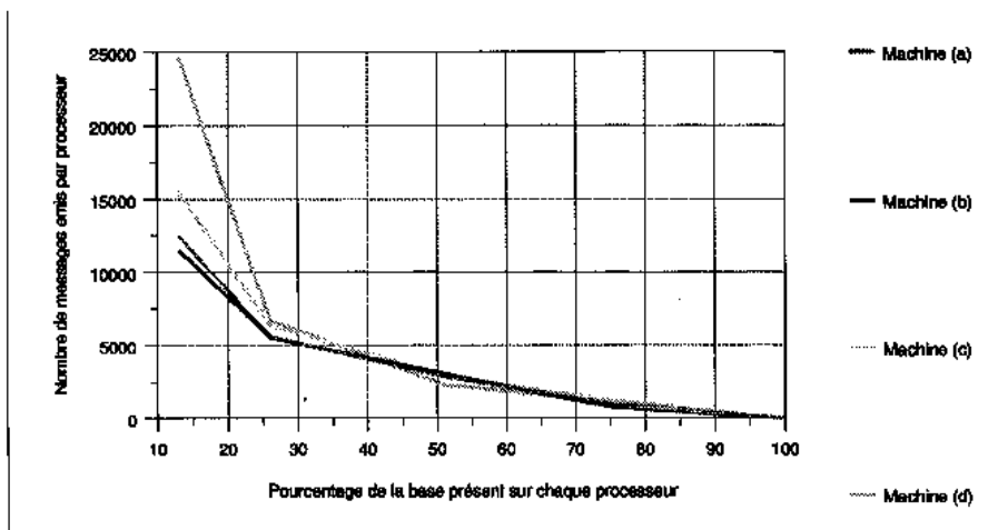
Figure 95 Nombre de messages émis sur les différentes machines
