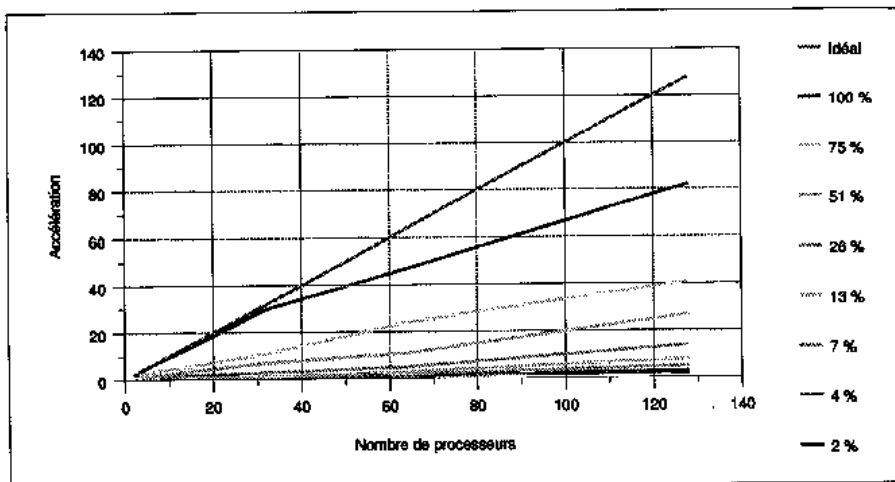
Figure 64 Accélération pour une distribution donnée en fonction du nombre de processeurs pour l'image M5.
