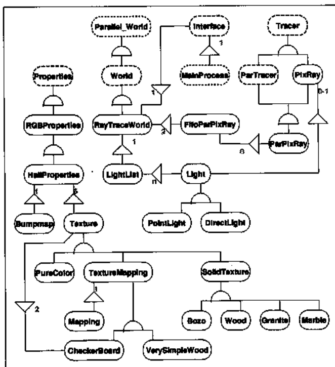
Figure 107 Diagramme objet du module optique
