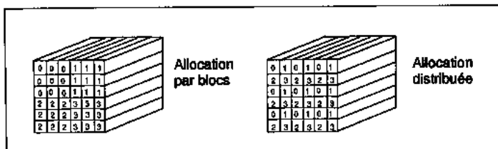
Figure 30 Allocation distribuée et allocation par blocs
