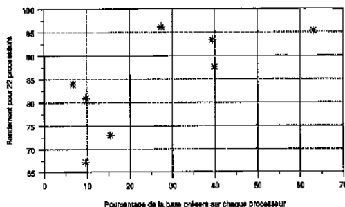
Figure 36 Rendement pour 22 processeurs sur différentes images en fonction du pourcentage de la base présent sur chaque processeur
