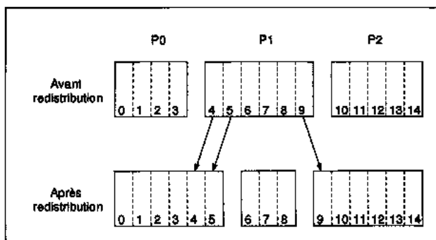
Figure 40 Redistribution de l'image
