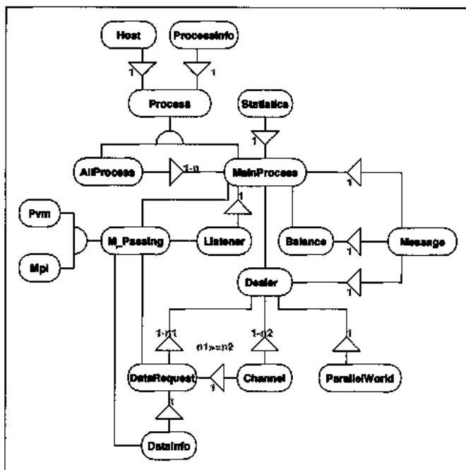
Figure 105 Diagramme objet du noyau parallèle
