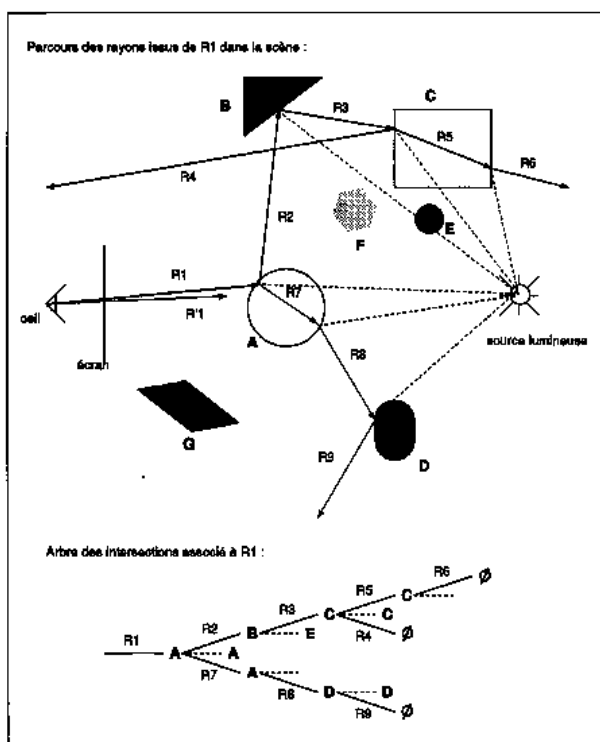
Figure 4 Arbre des intersections d'un rayon
