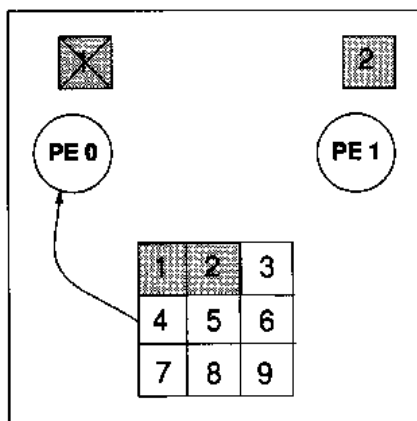
Figure 26 Distribution dynamique cohérente
